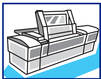
Bitmap data
